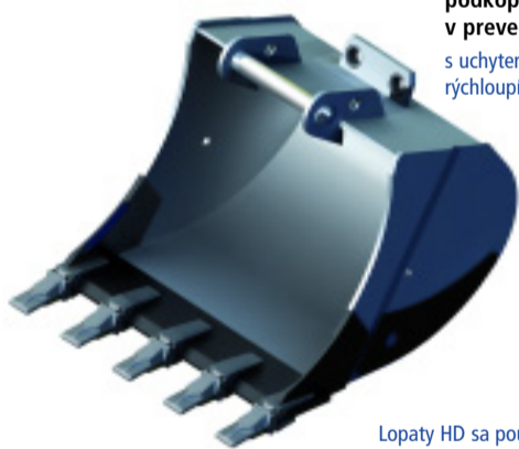
podkopová lopata KM65 v prevedení HD s uchytением pre rýchlopínač Verachtert CW
