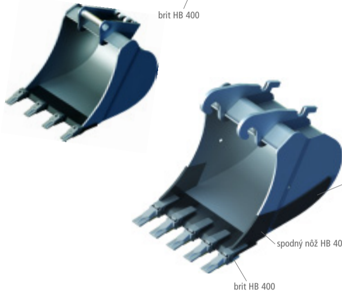
prevedenie s uchytением pre rýchlopínač Verachtert CW
